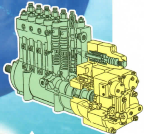
▲コマツ自社開発の電子ガバナ 可変噴射タイミング機構内蔵 高圧噴射ポンプ KP-21
